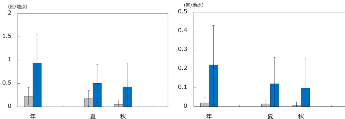
図3-7 短時間強雨の年・季節別発生回数の変化（青森県） （左：1時間降水量30mm以上、右：1時間降水量50mm以上）
