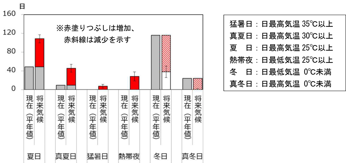
図3-4 階級別日数の変化 (青森県)
