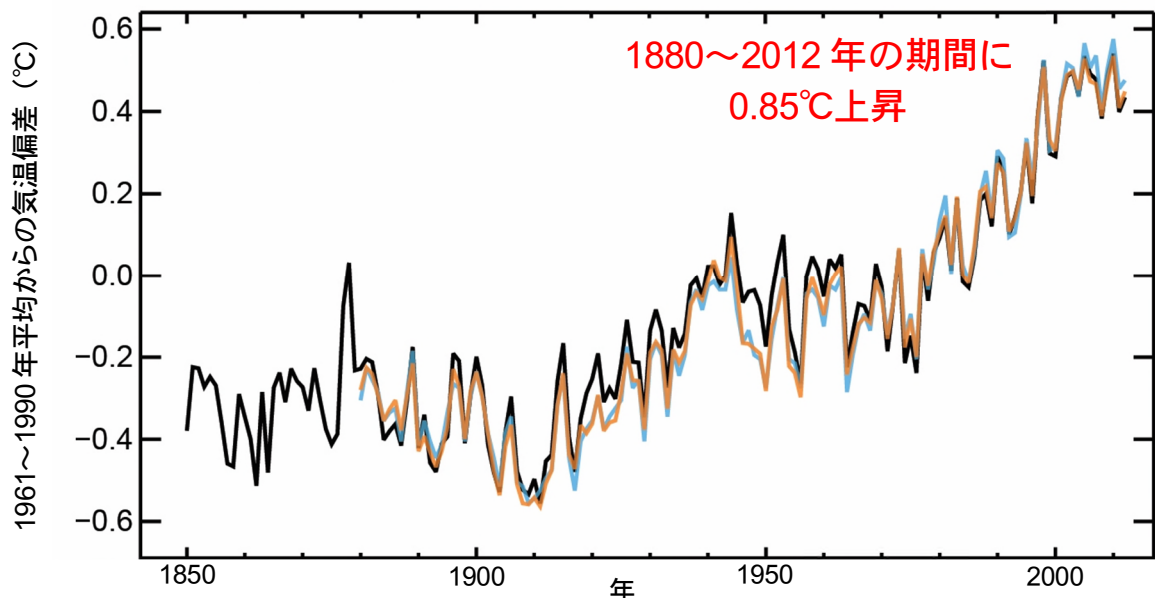
図1-3 世界の年平均気温の経年変化 (年平均)
