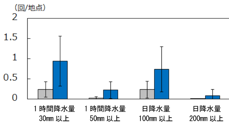
図3-8 短時間強雨（1時間降水量30mm以上、1時間降水量50mm以上）と大雨（日降水量100mm以上、200mm以上）の年間発生件数の変化（青森県）
