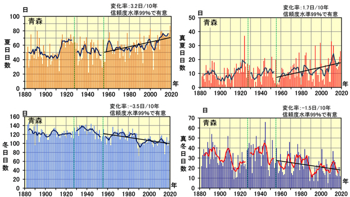
図3-2 夏日、真夏日、冬日、真冬日日数の推移（青森市）
