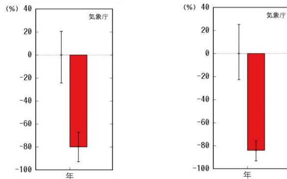
図3-11 年降雪量及び年最深積雪量の変化率（青森県） （左：年降雪量、右：年最深積雪）
