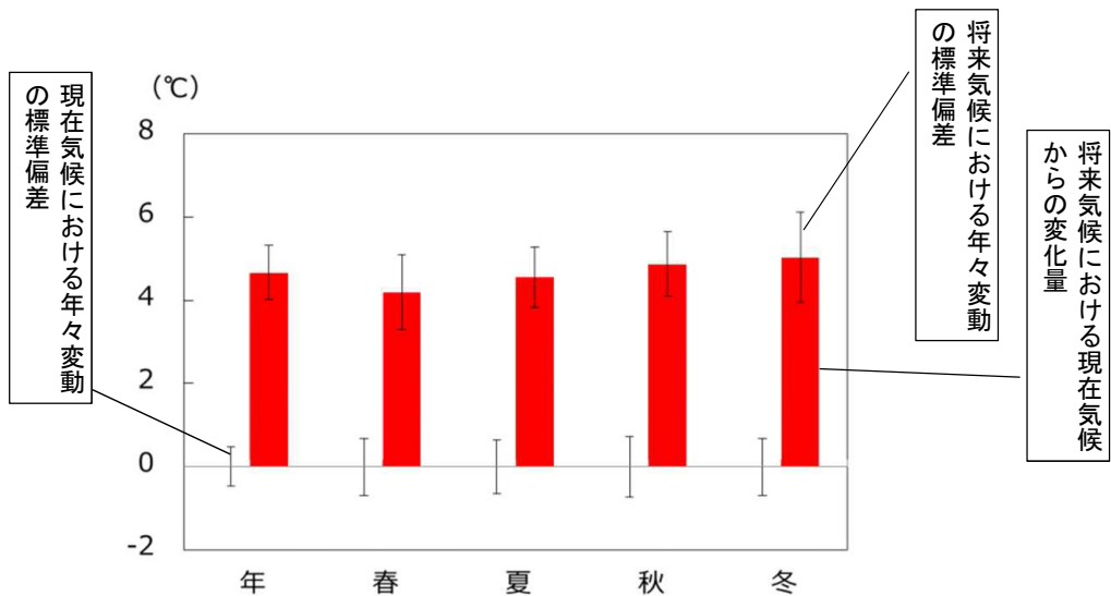
図3-3 年・季節別平均気温の変化 (青森県)
