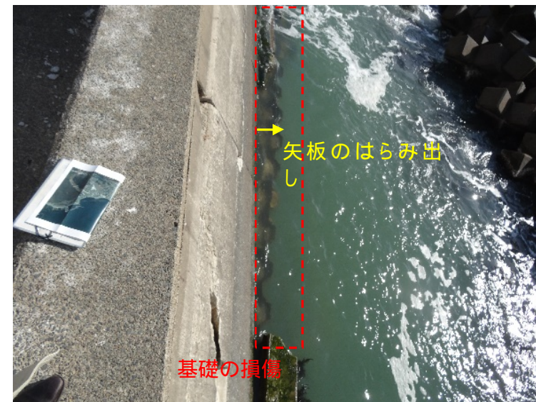
脇元海岸(五所川原市) 被災状況 - 基礎の損傷状況 -
