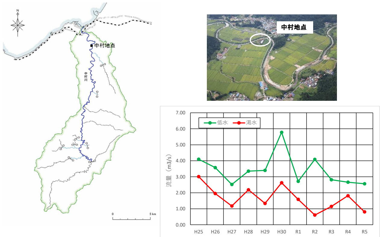
図 1-14 中村地点の低水流量と渇水流量
