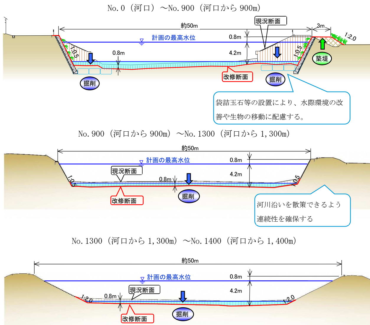
図 3-2 改修断面
