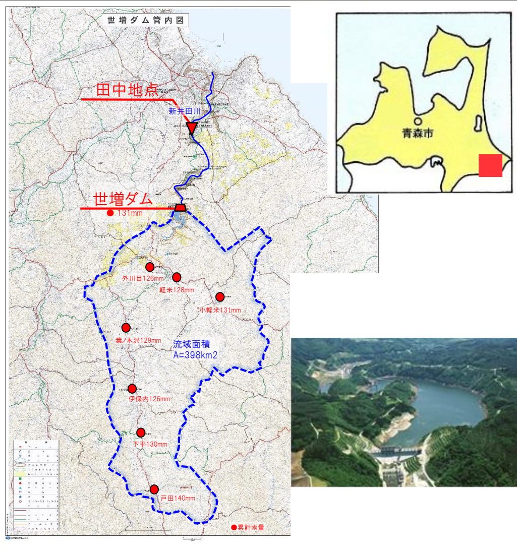
【世増ダム地点雨量】
