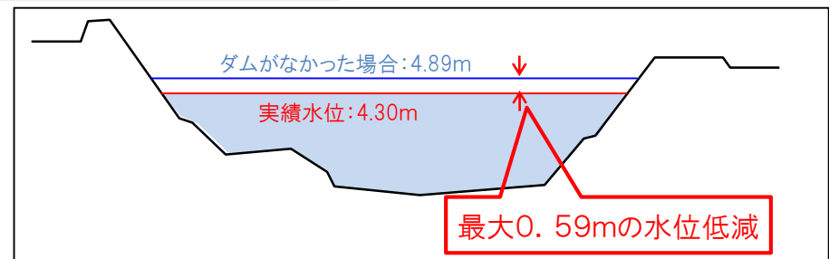
田中地点での水位低減効果
