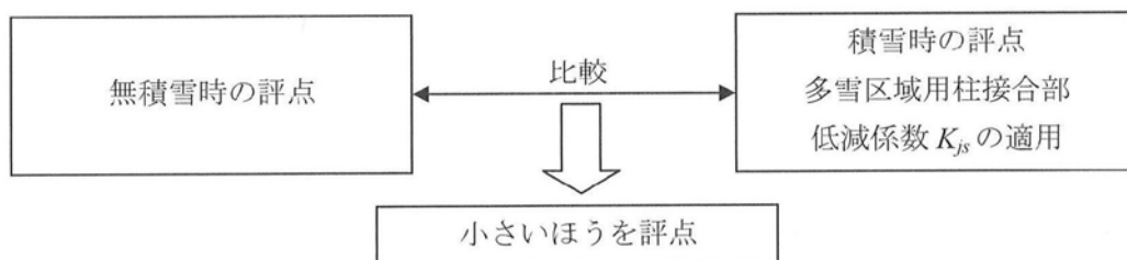
解図 3.2 多雪区域の耐震診断の流れ
