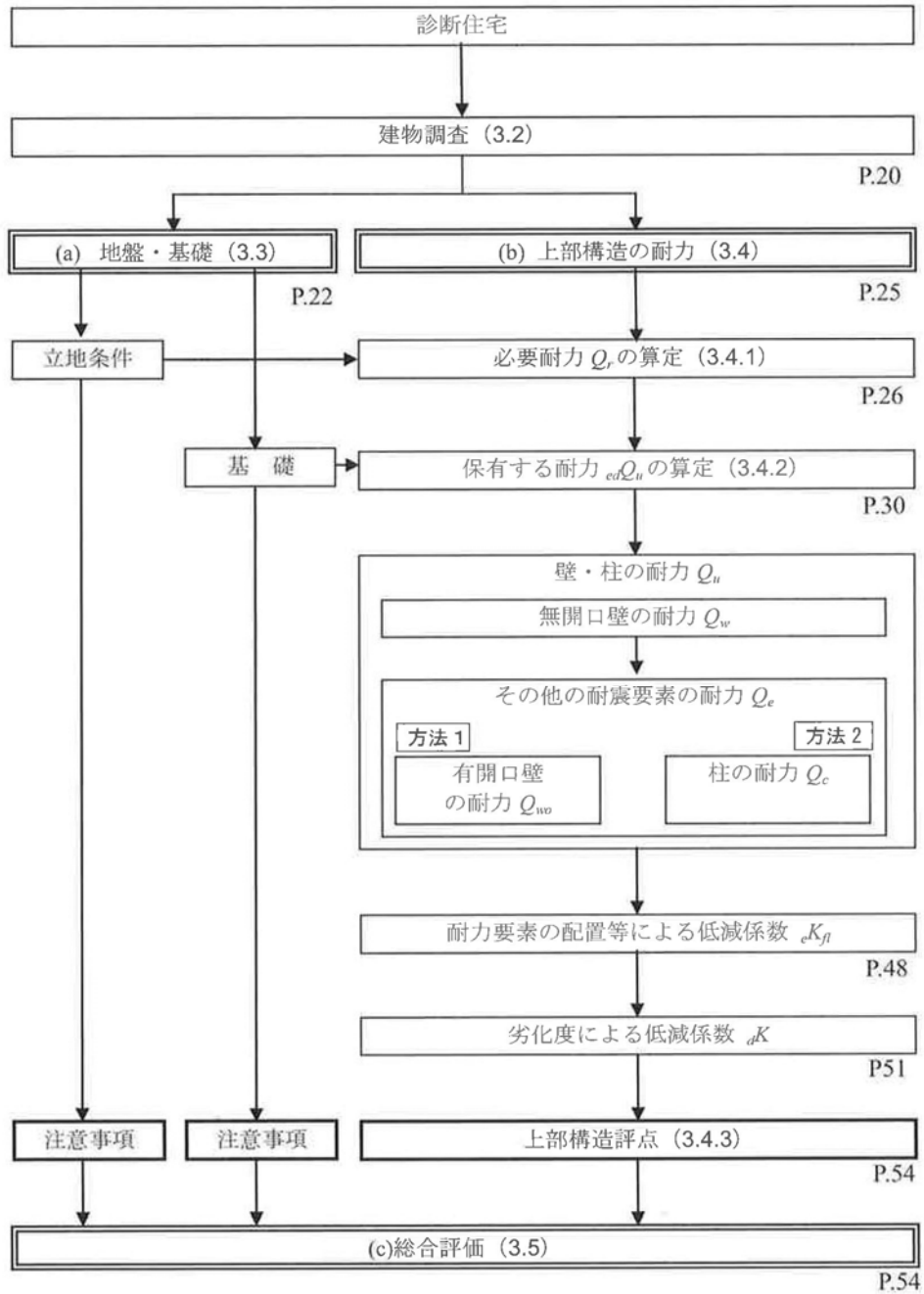
解図 3.1 一般診断の流れ
