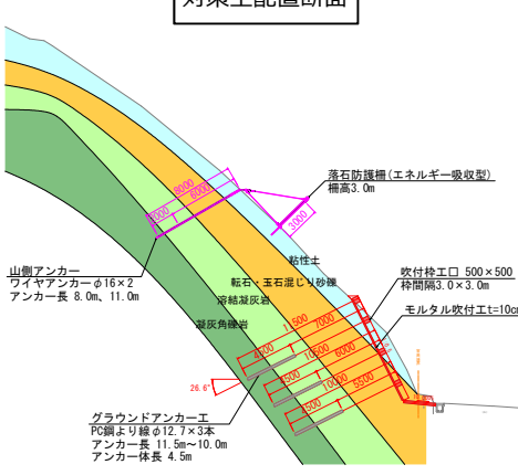
対策工配置断面
