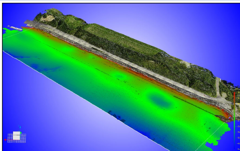
3次元点群測量データ
