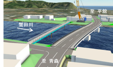
図-4 施工時イメージ(仮設歩道橋架設時)
