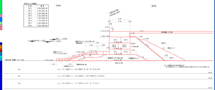
本設計護岸 標準断面図
