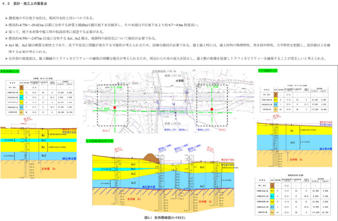
橋梁基礎の支持層及び基礎形式
