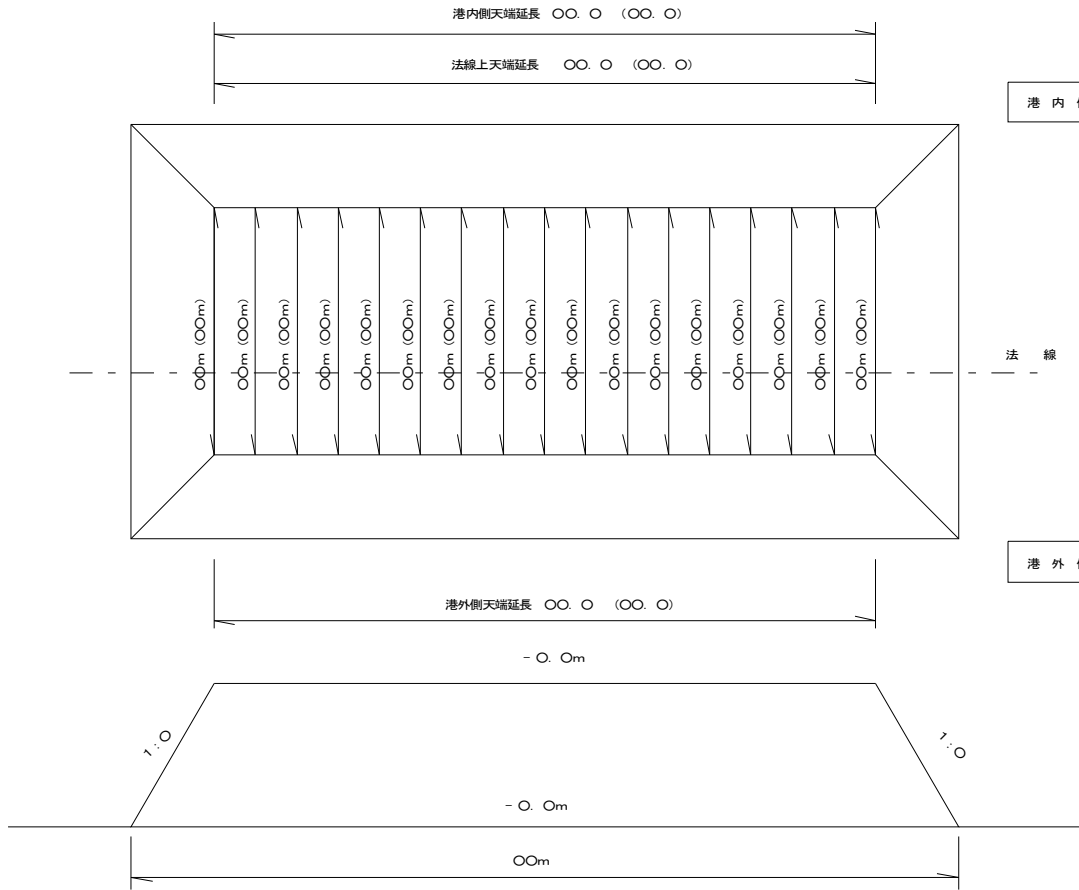
標準断面图
