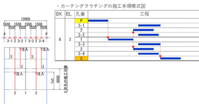
実施工を考慮した同時注入による工期短縮策
