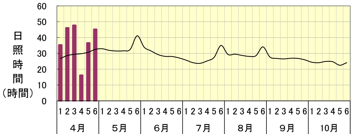
半旬別気象図・日照時間(青森:令和6年)
