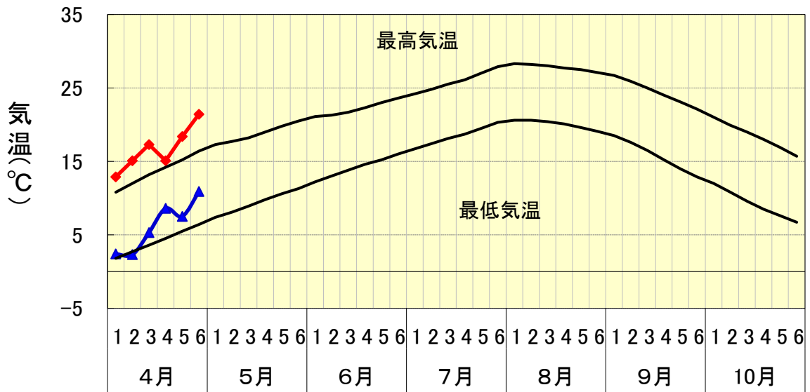
半旬別気象図 最高気温・最低気温(青森:令和6年)
