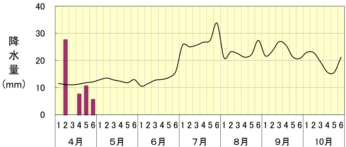
半旬別気象図・降水量(青森:令和6年)
