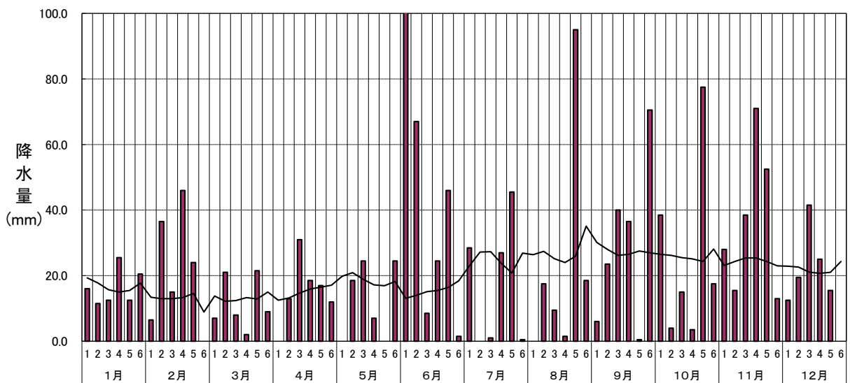
半旬別気象図 降水量(深浦:2017年)
