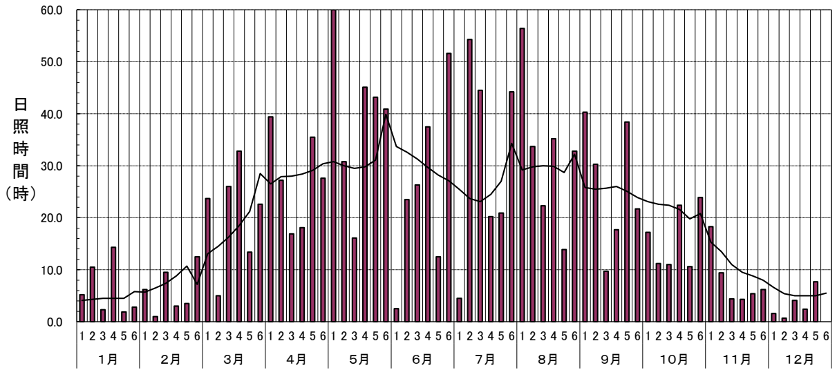
半旬別気象図 日照時間(深浦:2017年)
