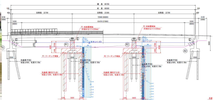
補強一般図
