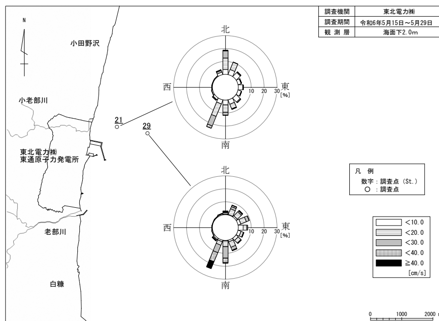
圖一3.8 流向別流速出現頻度
