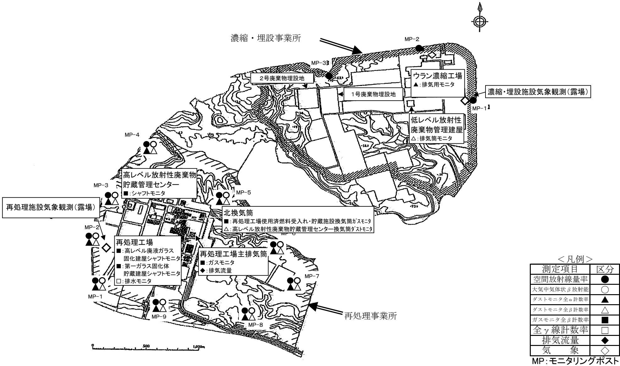
図3 日本原燃株式会社から提供を受ける周辺監視区域内の測定場所
