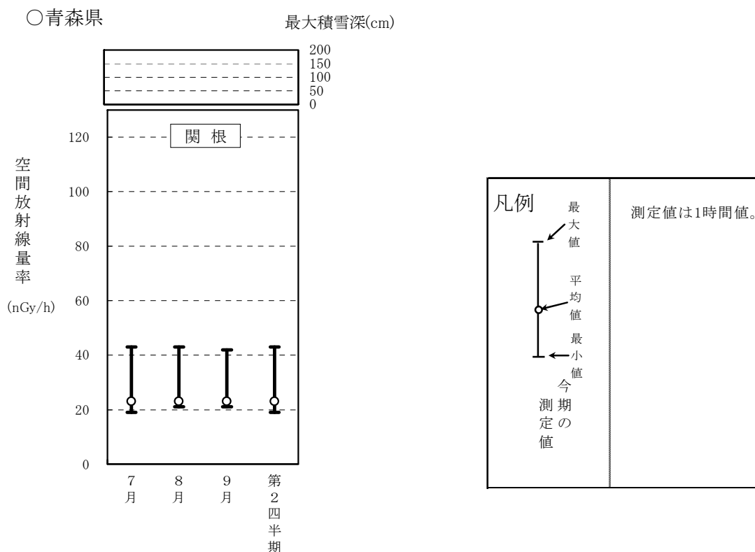
図2-2 RPLDによる積算線量測定結果 (注1)
