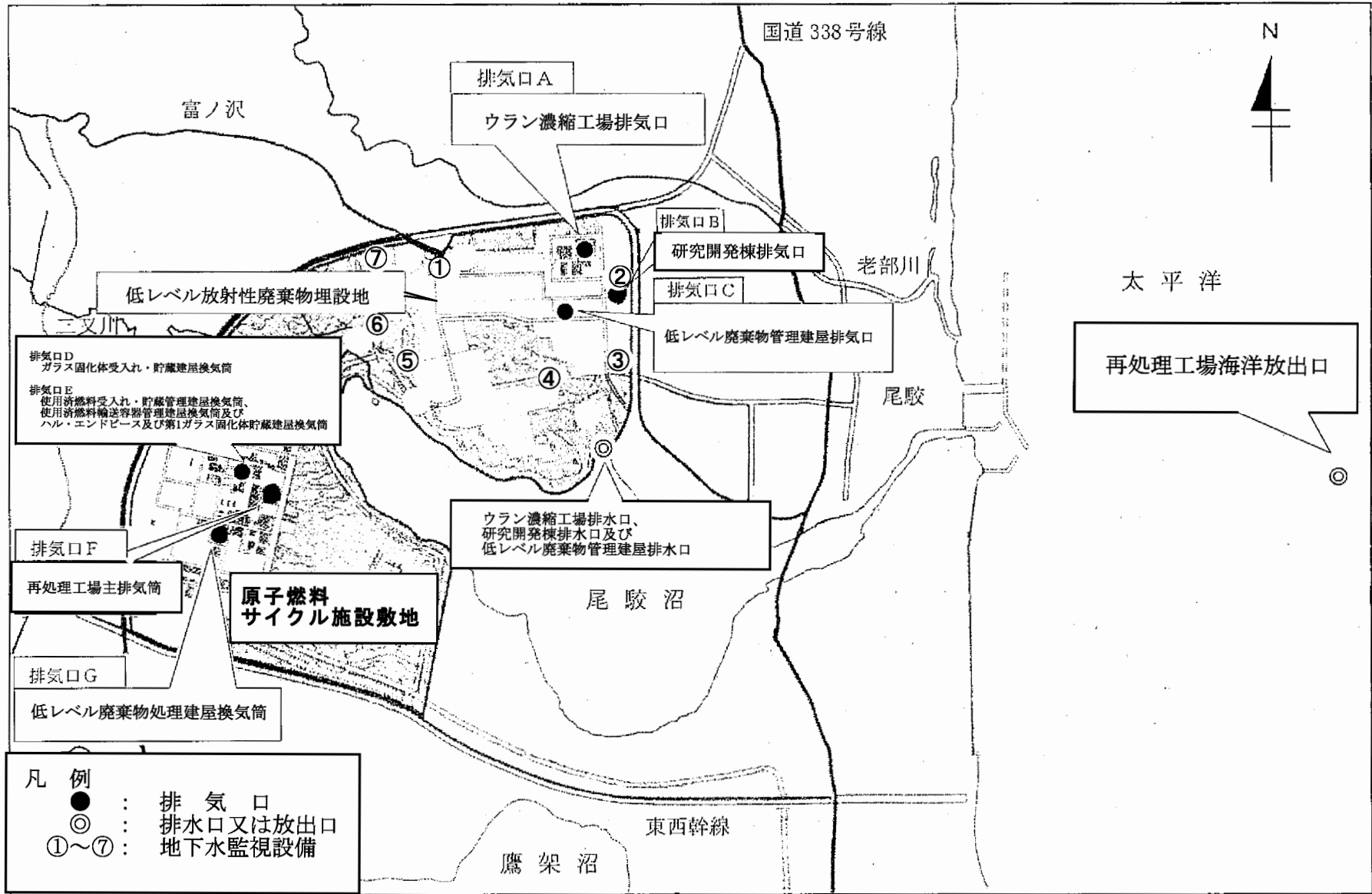
図 原子燃料サイクル施設の排気口、排水口、放出口及び地下水監視設備位置図
