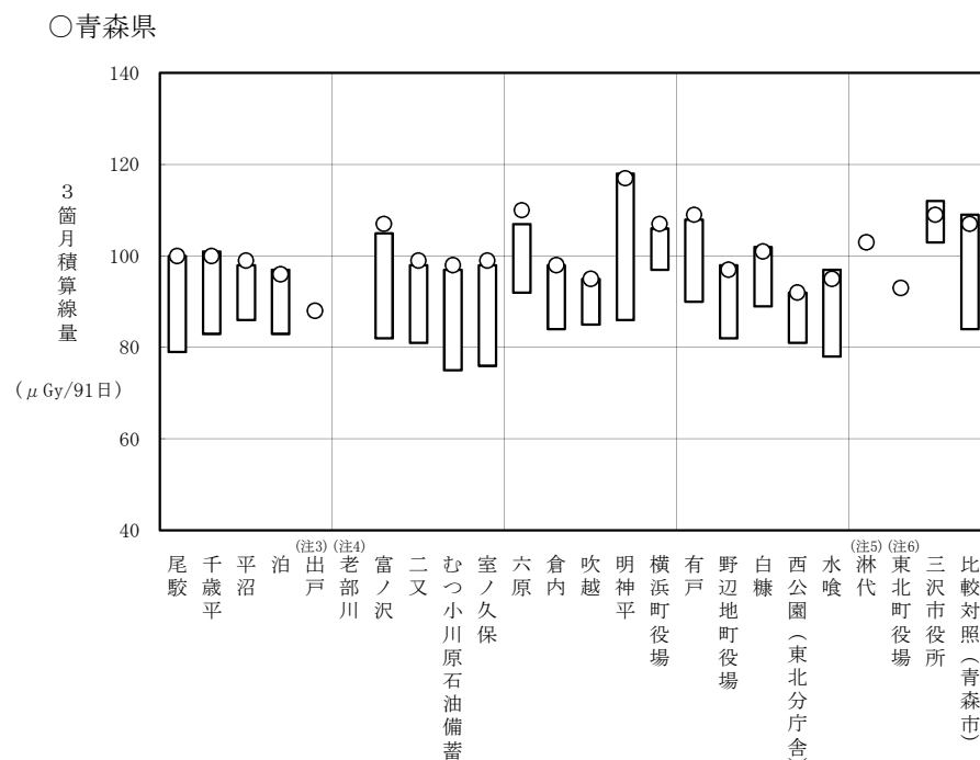
図2-4 RPLDによる積算線量測定結果 (注1)
