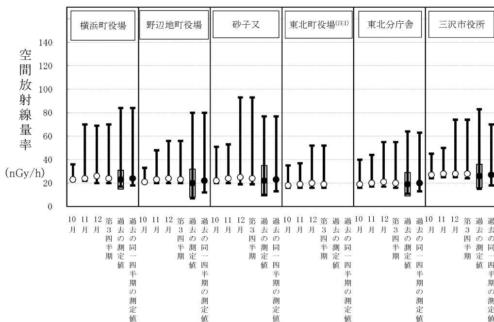
図 2-2 モニタリングポストによる空間放射線量率（NaI）測定結果
