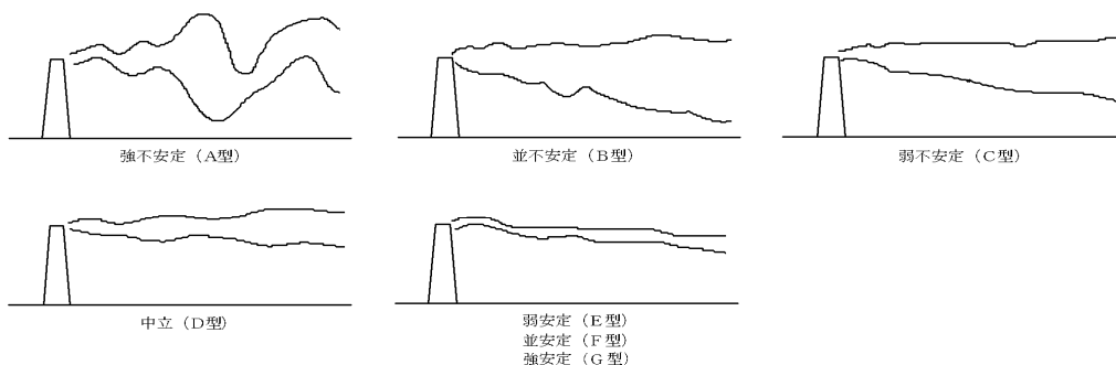
大気安定度と煙の型との模式図
