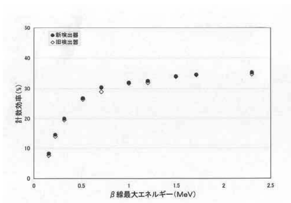
図2 \beta 線エネルギーと計数効率の関係
