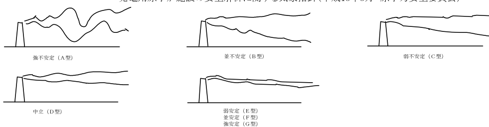
大気安定度と煙の型との模式
