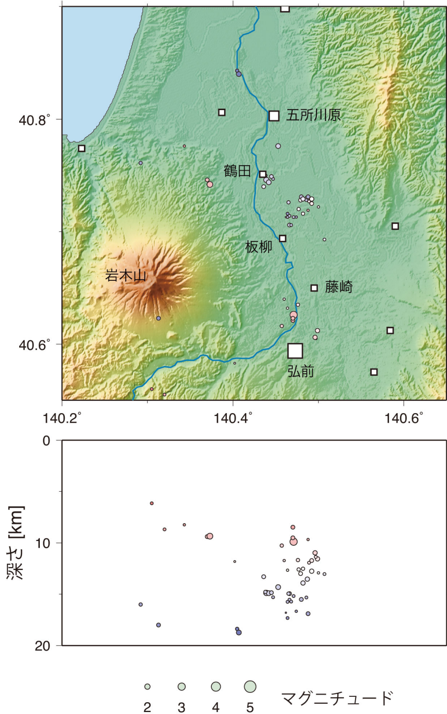
第2図 平成25年度に岩木山周辺で発生した地震の震源分布。下段は地震の深さ分布を東西断面図に投影したもの。丸の色は震源の深さを表し、丸の大きさはマグニチュードを表す。
