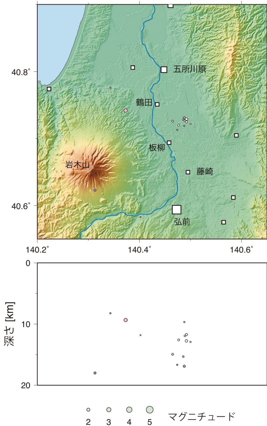
第7図 平成26年(2014年)1月～3月の期間に岩木山周辺で発生した地震の震源分布. 下段は地震の深さ分布を東西断面図に投影したもの. 丸の色は震源の深さを表し, 丸の大きさはマグニチュードを表す.
