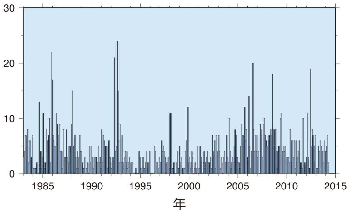
第1図 岩木山周辺で発生した地震の月別発生数. 上段は昭和48年(1973年)1月~平成26年(2014年)3月, 下段は昭和58年(1983年)1月~平成26年(2014年)3月の期間の発生数を示す.
