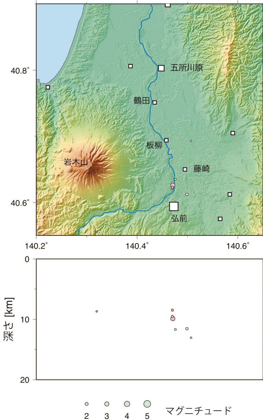
第5図 平成25年(2013年)7月～9月の期間に岩木山周辺で発生した地震の震源分布。下段は地震の深さ分布を東西断面図に投影したもの。丸の色は震源の深さを表し、丸の大きさはマグニチュードを表す。
