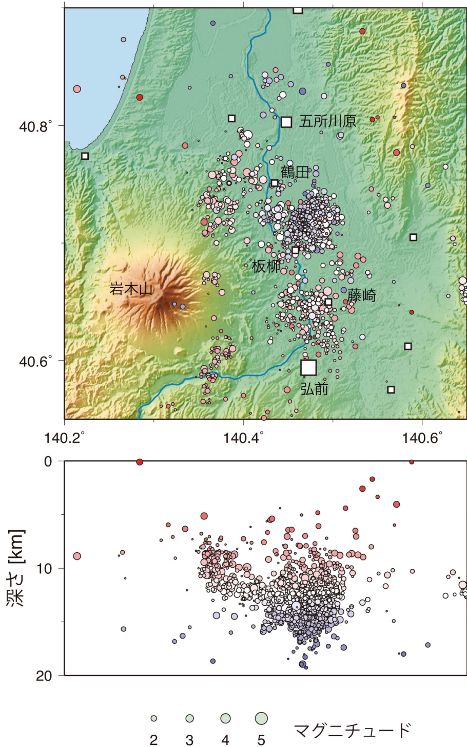
第3図 昭和58年(1983年)4月～平成25年(2013年)3月の期間に岩木山周辺で発生した地震の震源分布。下段は地震の深さ分布を東西断面図に投影したもの。丸の色は震源の深さを表し、丸の大きさはマグニチュードを表す。
