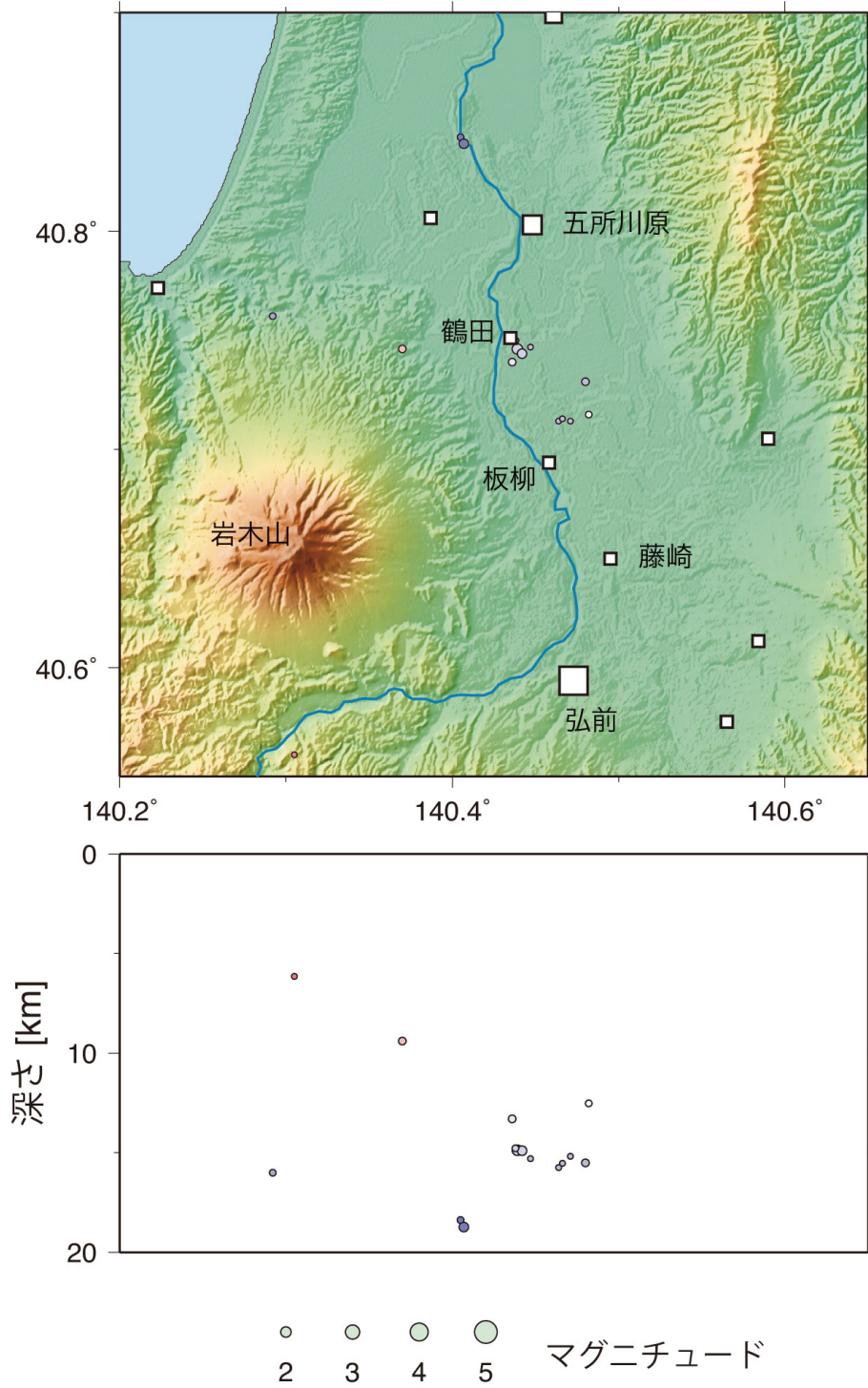
第4図 平成25年(2013年)4月～6月の期間に岩木山周辺で発生した地震の震源分布。下段は地震の深さ分布を東西断面図に投影したもの。丸の色は震源の深さを表し、丸の大きさはマグニチュードを表す。
