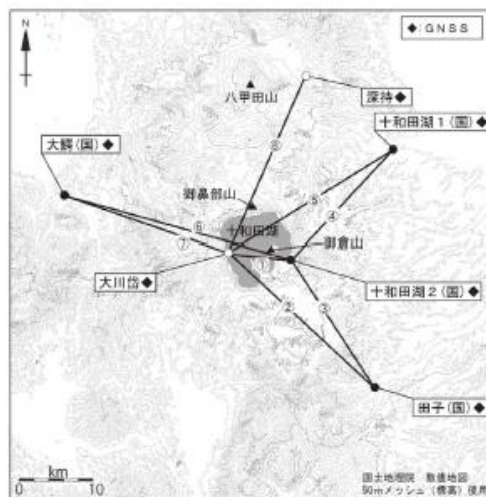
十和田 GNSS 観測点配置図
