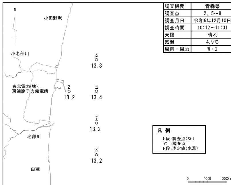
図－2.1 水温水平分布図（表層）
