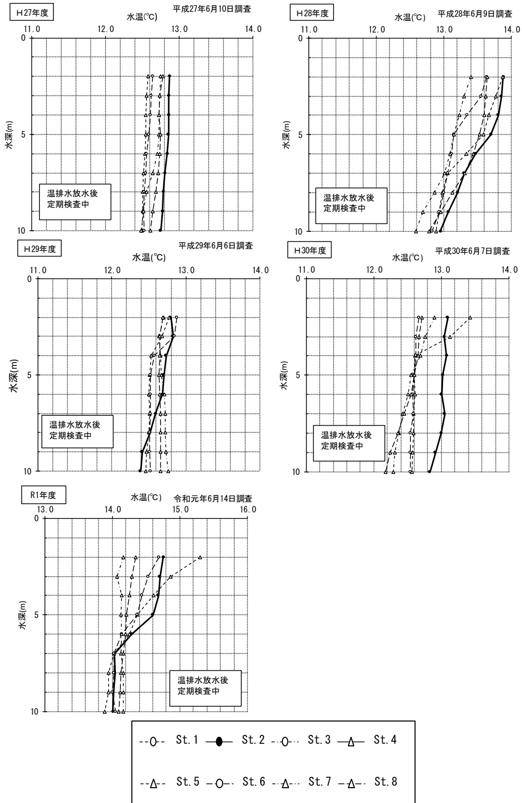
図-2.1 (3) 第1四半期水温鉛直分布
