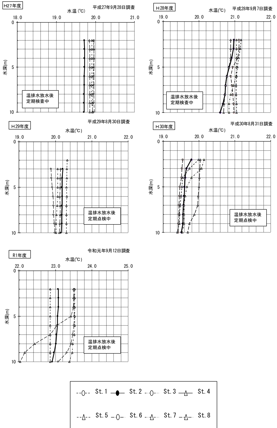
図-2.2 (3) 第2 四半期水温鉛直分布
