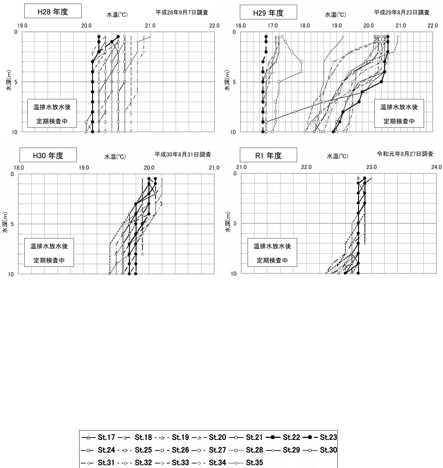
図-3.2(3) 第2四半期水温鉛直分布
