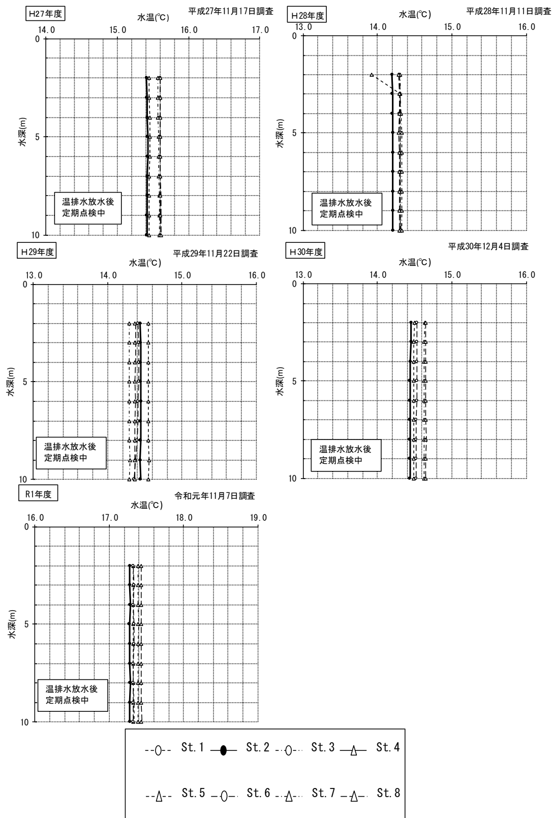
図-2.3 (3) 第3四半期水温鉛直分布
